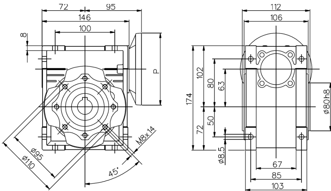
Выходной фланец и вал редуктора РС 63
