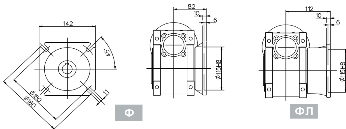
Выходной фланец и вал редуктора РС 63
