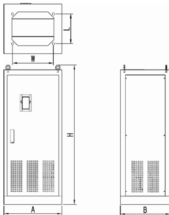
Металлический напольный шкаф
